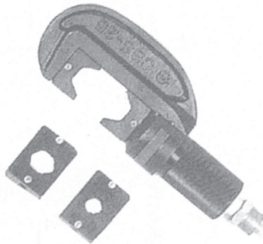
5 台製壓接工具(含13、20、25之模具)
