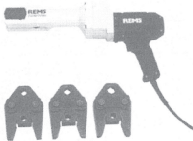
8 電動壓接工具(含13、20、25之模具)
