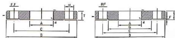
ANSI 300型 FLANGES
