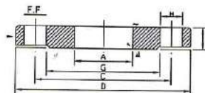
ANSI 125型 FLANGES
