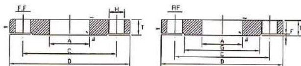
JIS 16kg/cm 2 型 FLANGES
