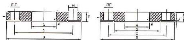
ANSI 150型 FLANGES
