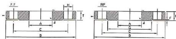
JIS 10kg/cm 2 型 FLANGES
