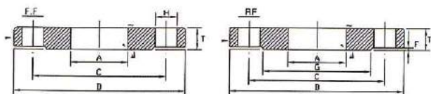
JIS 20kg/cm 2 型 FLANGES
