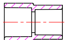
異徑直接頭 Red. COUPLING
