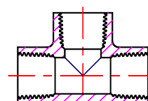
90°套銅內牙接頭 S*T
