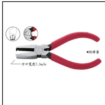
電子平嘴鉗
