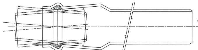
可撓性活套管簡圖
